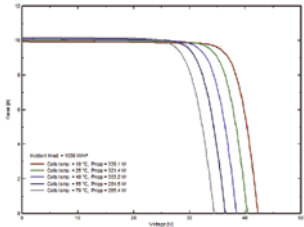
不同辐照度下I-V曲线 (SPP320M60S)
