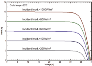
不同辐照度下I-V曲线 (SPP320M60S)
