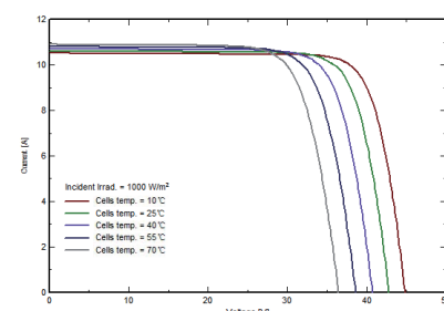
各動作温度条件の下にI-V曲線 (SPP365NHEH)
