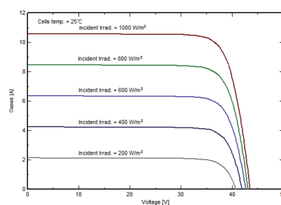
各日射強度条件の下にI-V曲線 (SPP365NHEH)
